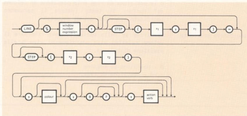
Figura 14-20 Istruzione LINE
